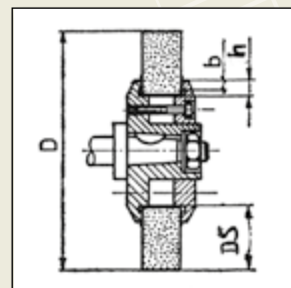
Rys. Oprawa kołnierzowa ściernic płaskich (wg PN / M-60625)
