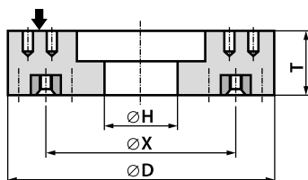
3601 - D x T x H - nr rysunku H \leq 0,67D
