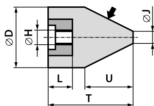
Ściernica walcowo - stożkowa z wkładką gwintową 19 - D / J × T / U - H × L
