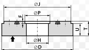
Ściernica tarczowa z wkładkami gwintowymi i wybraniem walcowym od strony mocującej 3603 - D \times T \times H - nr rysunku
