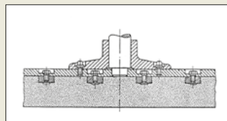
Rys. Ściernica przykręcona do tarczy nośnej; przykrecone do wrzeciona szlifierki
