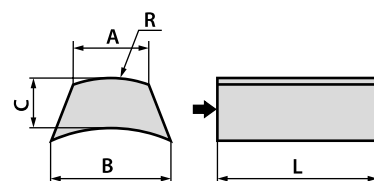
Segment pierścieniowy odwrótny 3124 - B / A \times C \times L - R...
