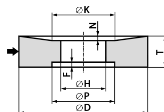
Ściernica z wybraniem stożkowym i walcowym z drugiej strony 22 - D / K × T / N × H - P... F...
