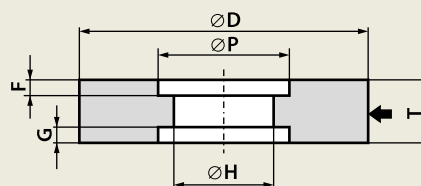
7 zarys - D x T x H - P...F...G...
