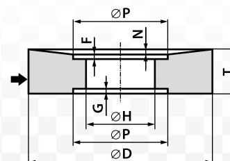
Ściernica z wybraniem stożkowo - walcowym i walcowym z drugiej strony 24 - D × T / N × H - P...F...G...
