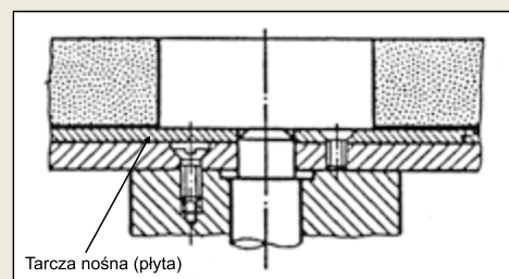
Rys. Ściernica przyklejona do tarczy nośnej; przykręcone do wrzeciona szlifierki.
