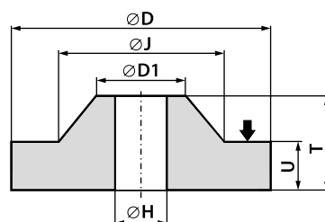
Ściernica o specjalnym kształcie do młynków pulpy warzywnej 3802 - D / J \times T / U \times H - nr rysunku
